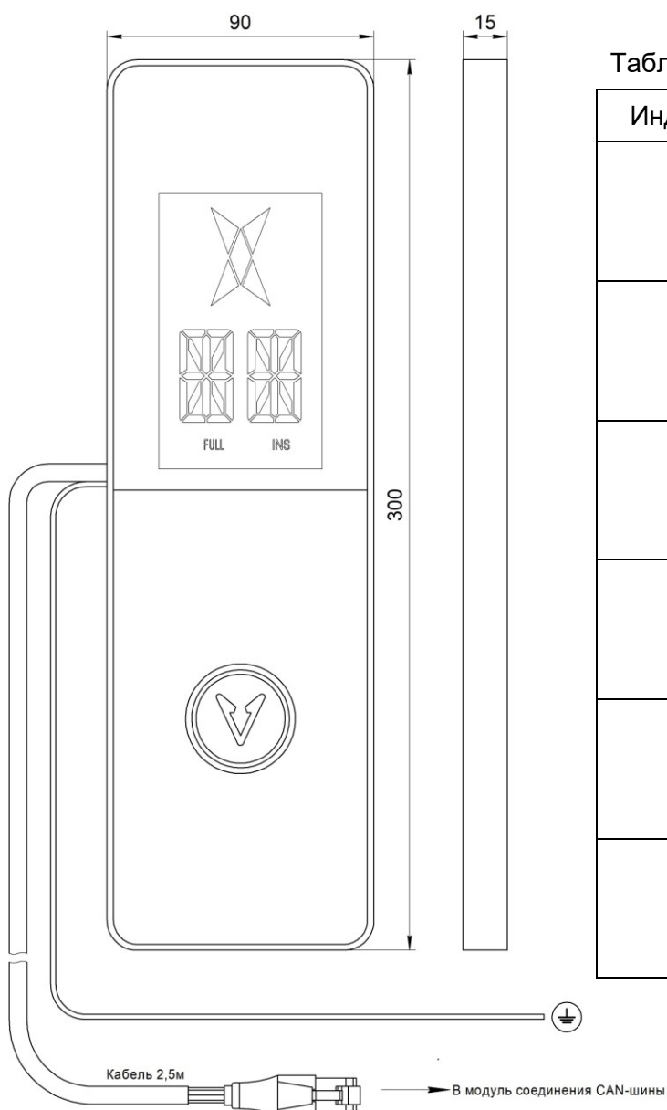
Рис.1 Внешний вид Вызывной пост ОНИКС (жгут RJ45) НШЕК.468381.117
